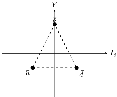
Anti-quarks 3^*
