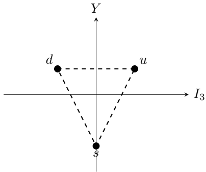
Quarks 3
